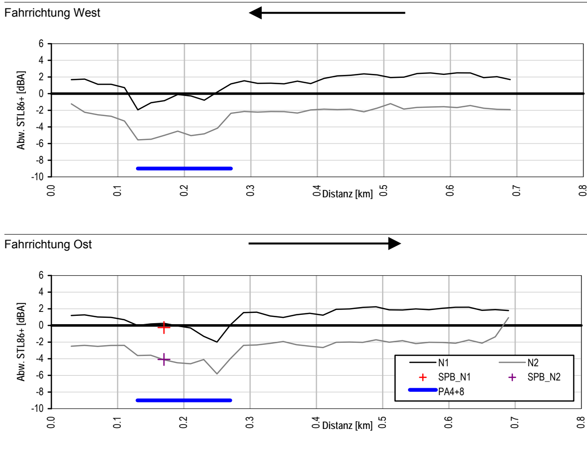
Abb. 7 CPX-Messung der Teststrecke in Kreuzlingen
